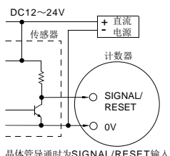
晶体管导通时为SIGNAL/RESET输入
